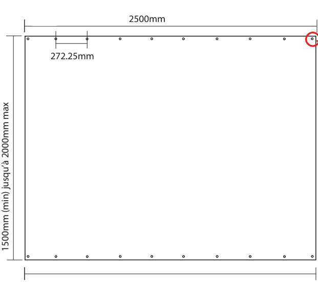
Dimensions du visuel et positionnement des oeillets
