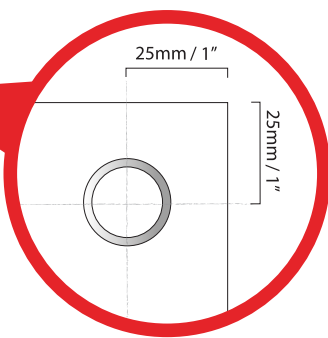
Positionnement des oeillets
